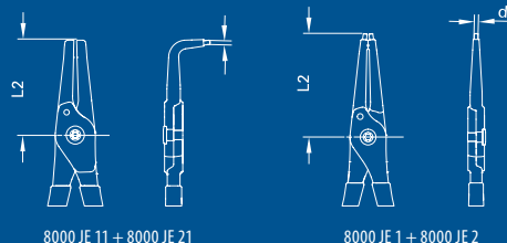
8000 JE 11 + 8000 JE 21
