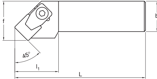
CSSNR/L.....12S
