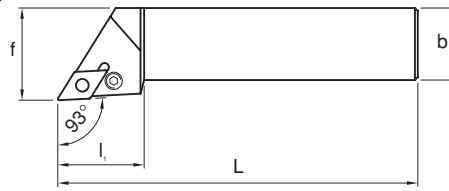
PDJN 93°
