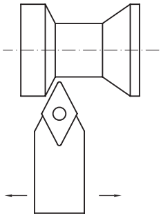
DDNN 63°
