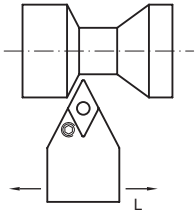
PDNN 93°
